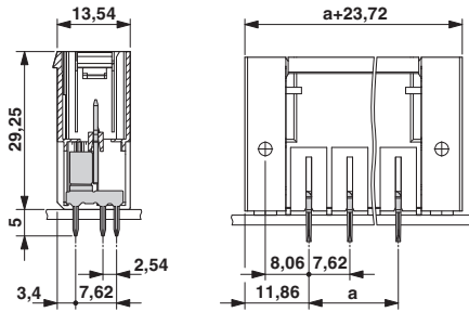
外形寸法
