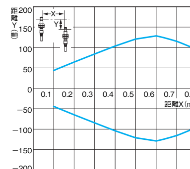
形E3T-CT2□S(上下方向)
