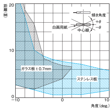
形E3T-FL2□ (上下方向)
