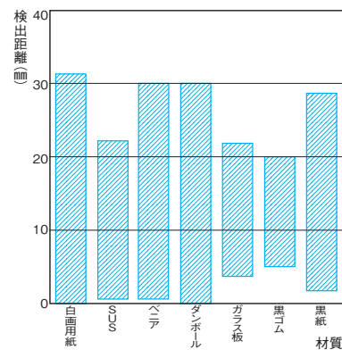
形E3T-FL2□
