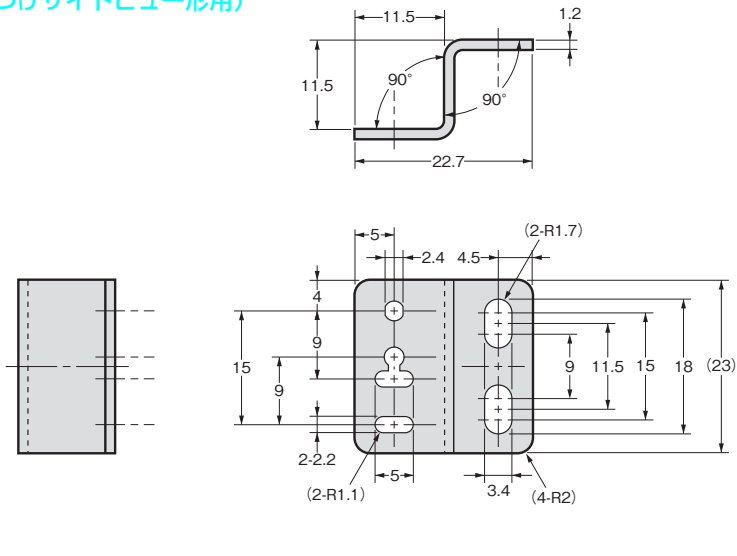
取り付け金具装着時 (形E3T-ST11の例)
