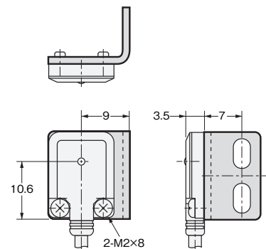
取り付け金具装着時 (形E3T-FT11の例)
