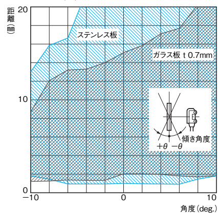
形E3T-SL2□(M) (上下方向)
