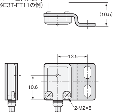
取り付け金具装着時 (形E3T-FT11の例)
