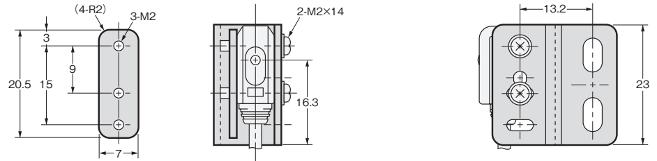
取り付け金具装着時 (形E3T-ST11の例)
