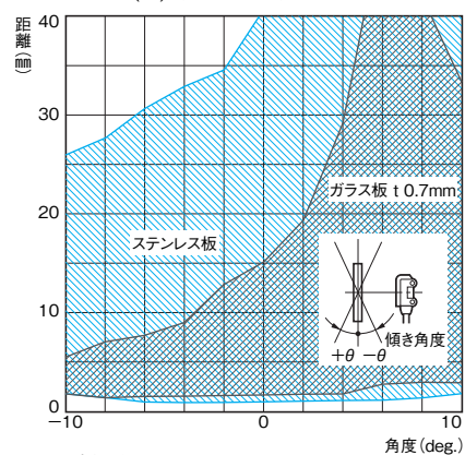
形E3T-FL1□ (上下方向)
