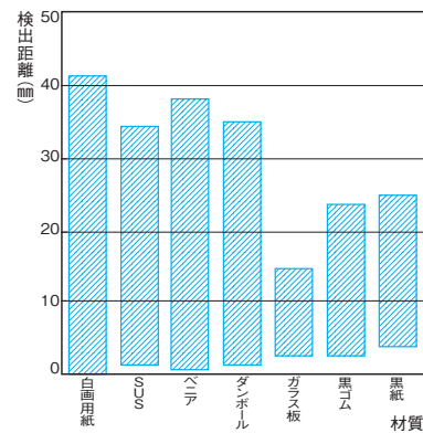
形E3T-SL2□(M)
