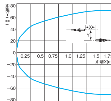
形E3T-CT1□
