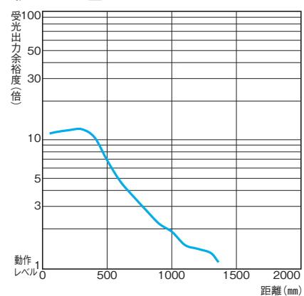
形E3T-ST2□F
