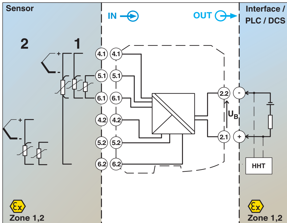
结构框图
