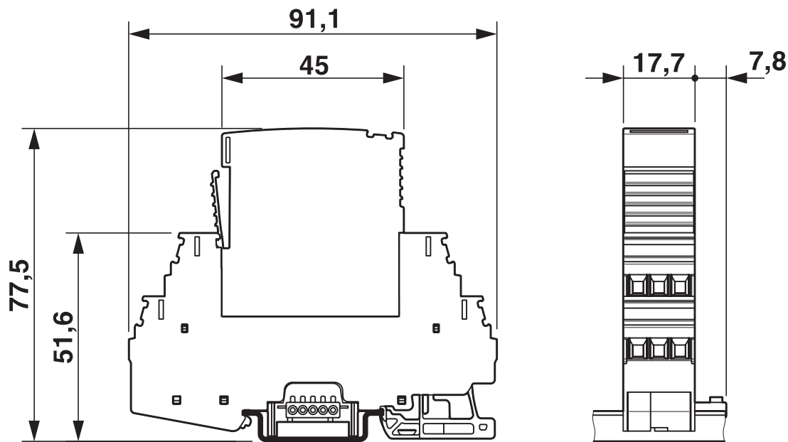
尺寸图
