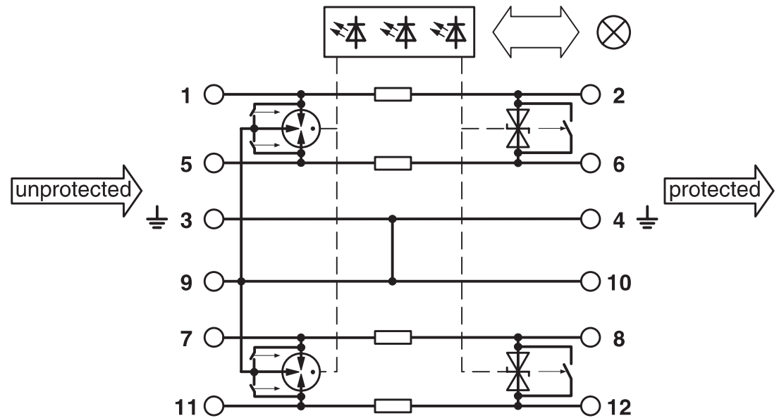
电路图
