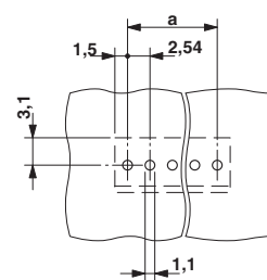
Dima di foratura
