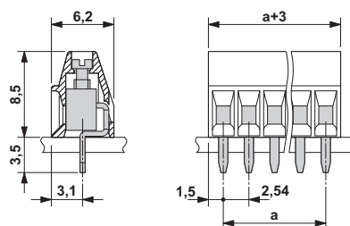
Disegno quotato
