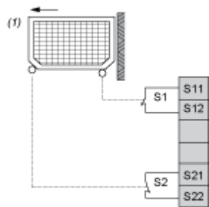
(1) 防护装置
