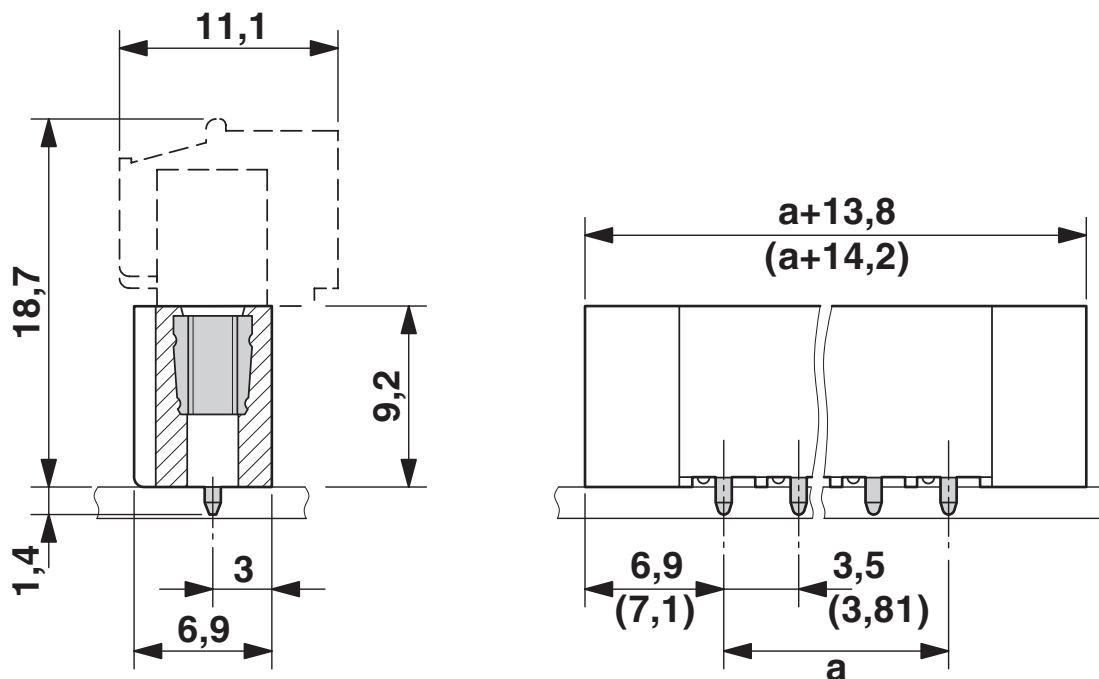
Maßzeichnung
