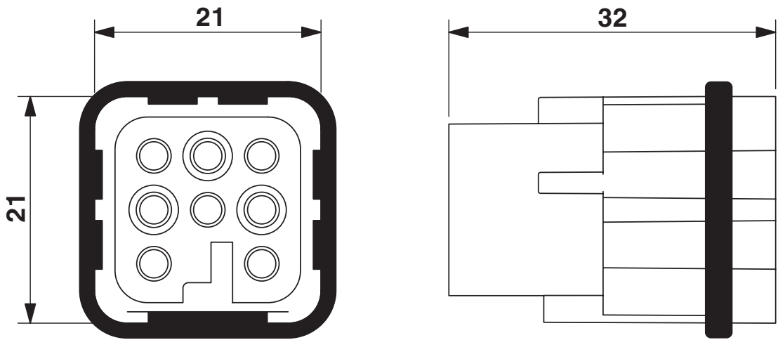
尺寸图
