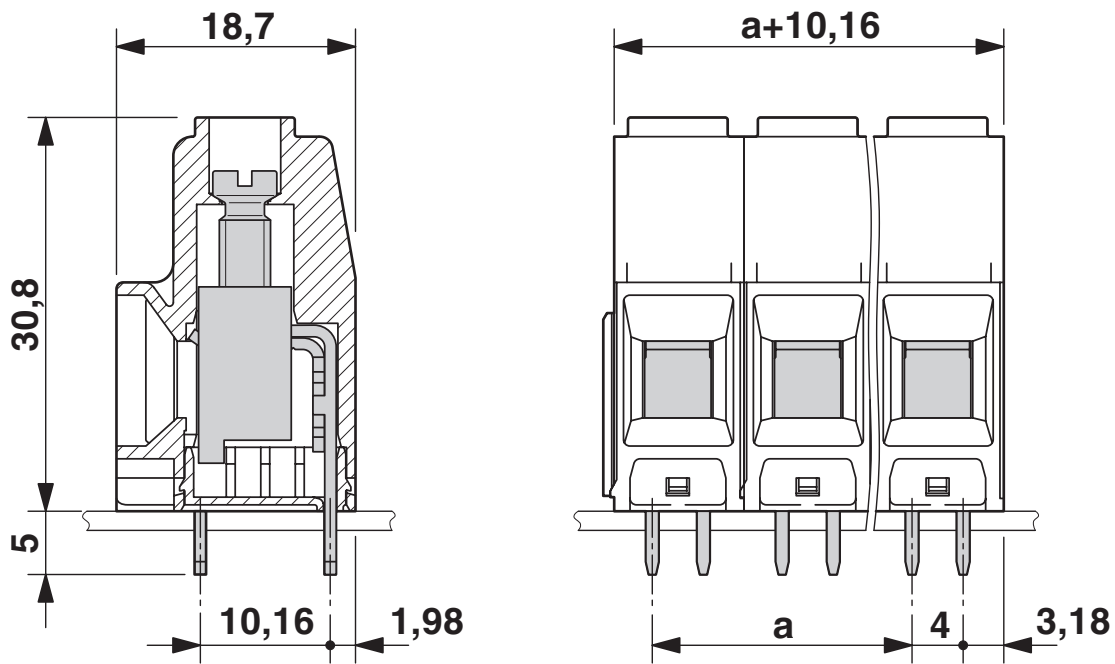
图为3位连接器的尺寸图
