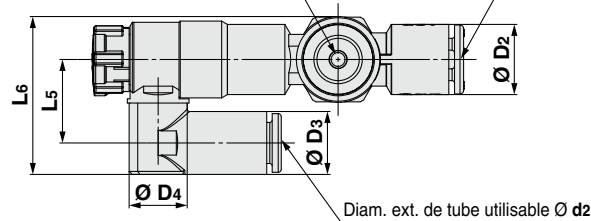
Bouton d'échappement de la pression résiduelle Ø D1
