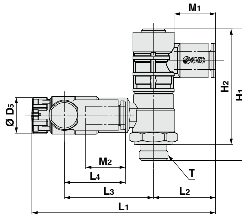
Modèle avec fonction d'échappement de la pression résiduelle
