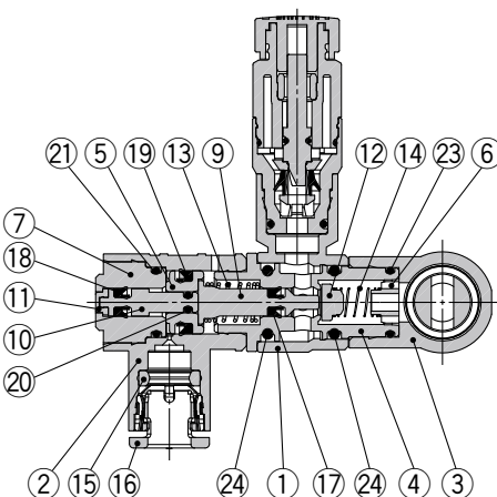
Modèle avec fonction d'échappement de la pression résiduelle
