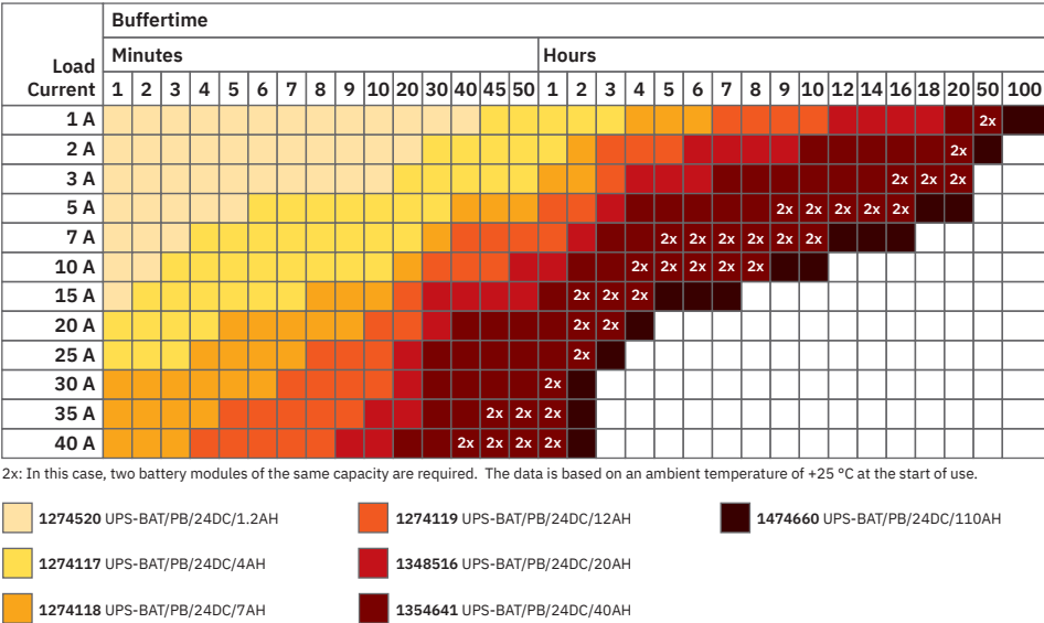
用于铅电池模块的QUINT DC UPS缓冲时间
