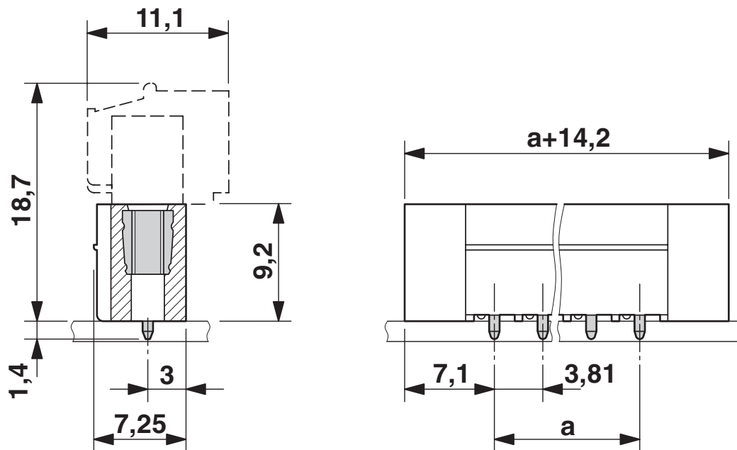
尺寸图
