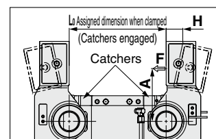
S-type arms
