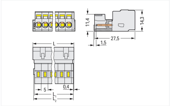
Dimensions en mm L = (\text{nombre pôles} - 1) \times \text{pas} + 8,2 \text{ mm} L2 = L - 1,7 \text{ mm} L3 = L - 1,2 \text{ mm}
