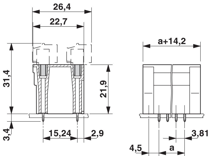
尺寸图
