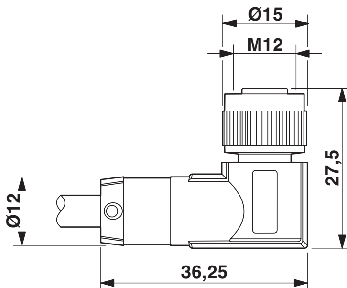
尺寸图
