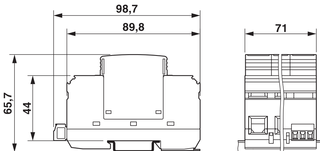
尺寸图
