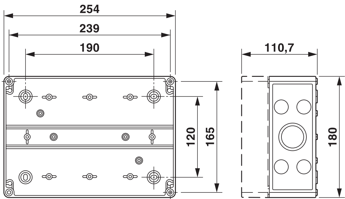
尺寸图
