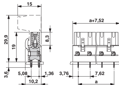
外形寸法
