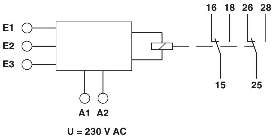
结构框图
