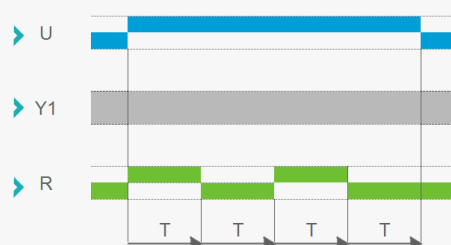
Funzione H: Temporizzazione alla messa sotto tensione
