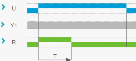
Funzione Ht: Temporizzazione alla messa sotto tensione totalizzatore A
