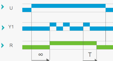
Funzione N: Watchdog
