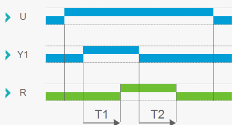
Funzione At: Totalizzatore A
