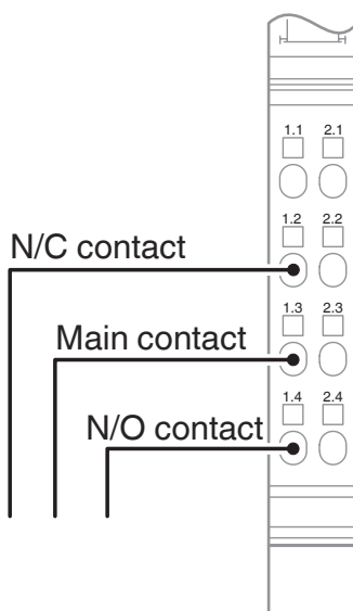
Anschlusszeichnung
