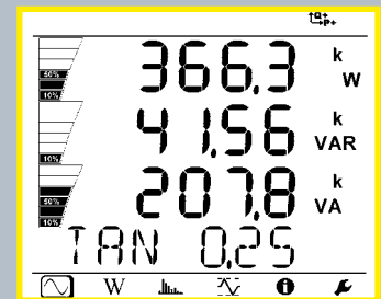
Leistung/Tan
