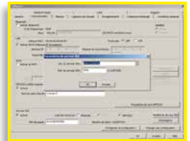
Konfiguration des IRD-Servers
