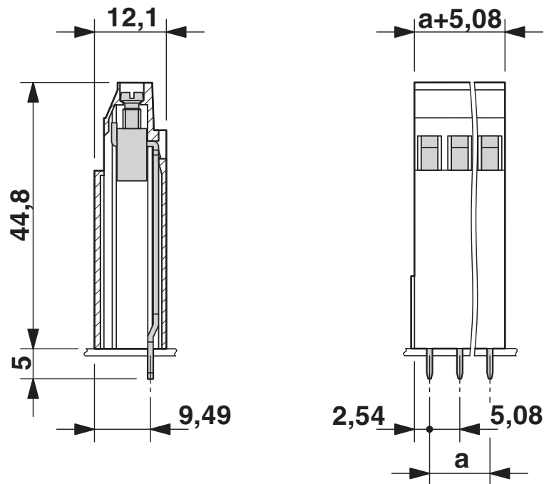
尺寸图
