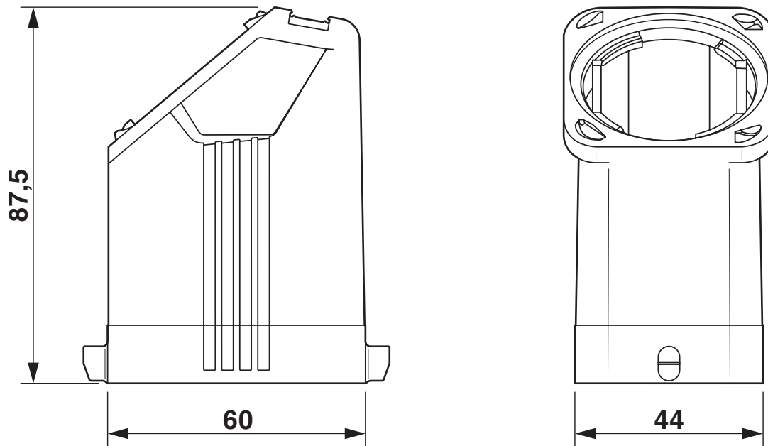
Maßzeichnung
