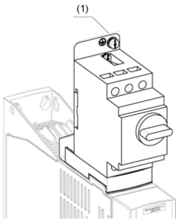
(1) 接地螺钉 ( HS 型 2 - 5x12 )
