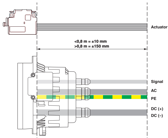
尺寸图
