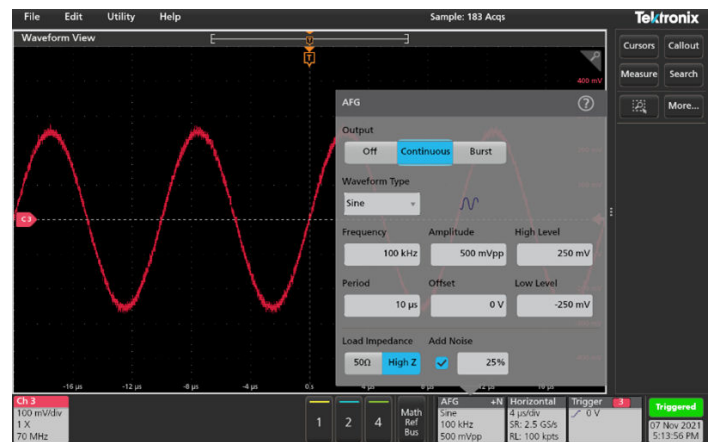
Ajustes flexibles de salidas AFG. En este caso de prueba, el 25 % del ruido se añadió al seno
