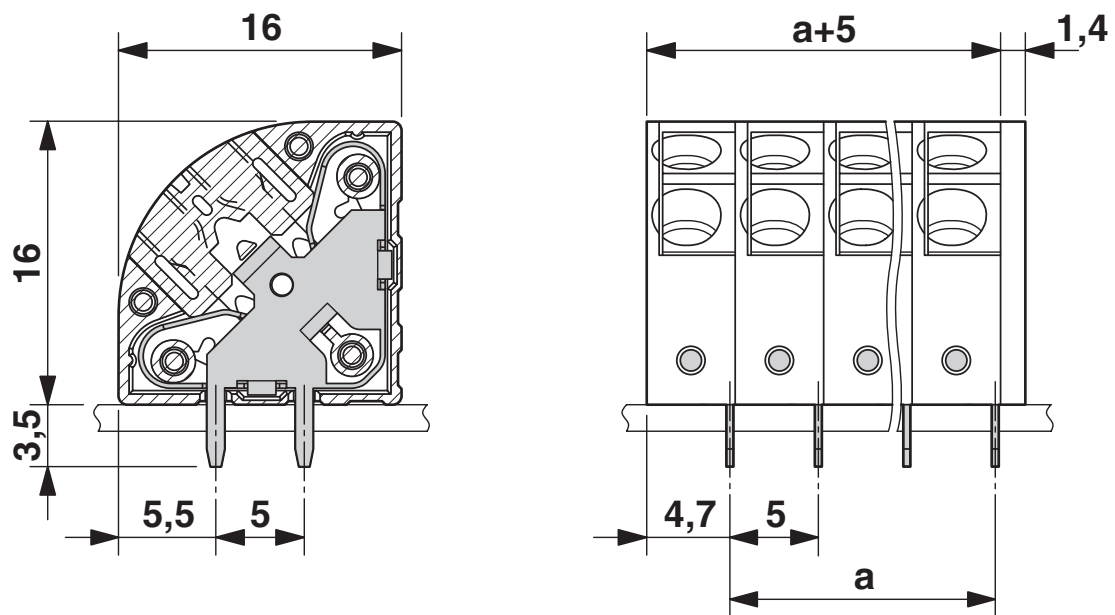
尺寸图
