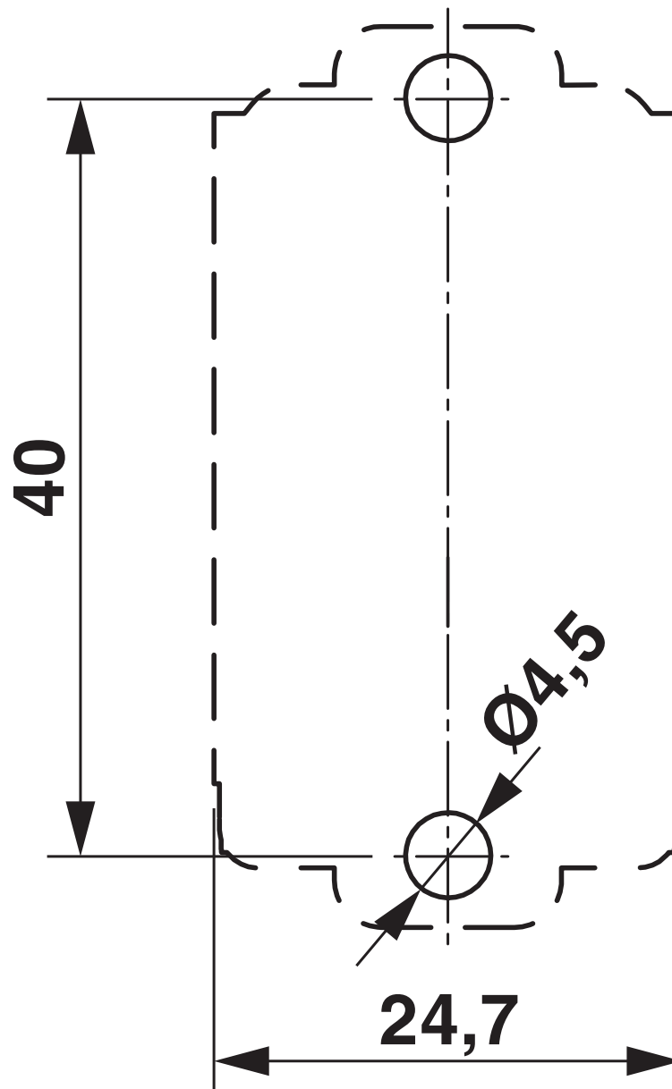
开孔图/焊盘环宽
