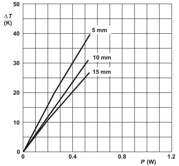
安装后导线端 (焊接点) 温差 (ΔT) 与不同导线长度耗散功率的函数
