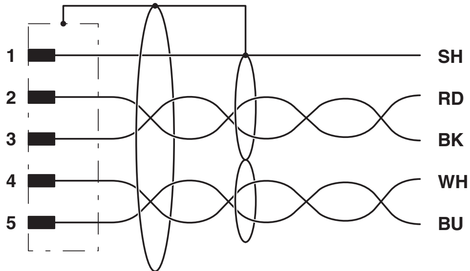
Schaltplan
