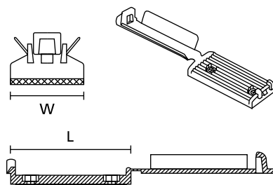
Embases pour câbles plats série FKH
