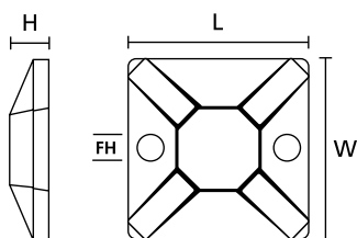
Embases de fixation MB3APT-MB5APT
