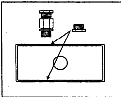
Fig. 1 : Cable Gland Positions
