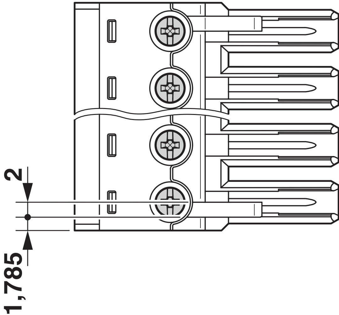
尺寸图
