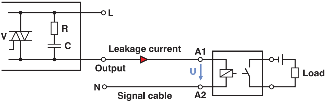
应用图
