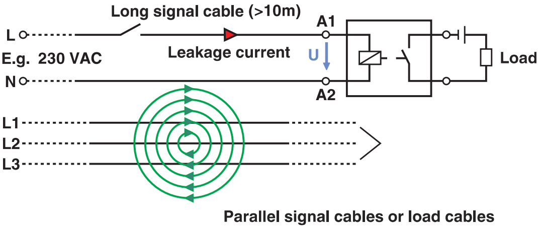
应用图
