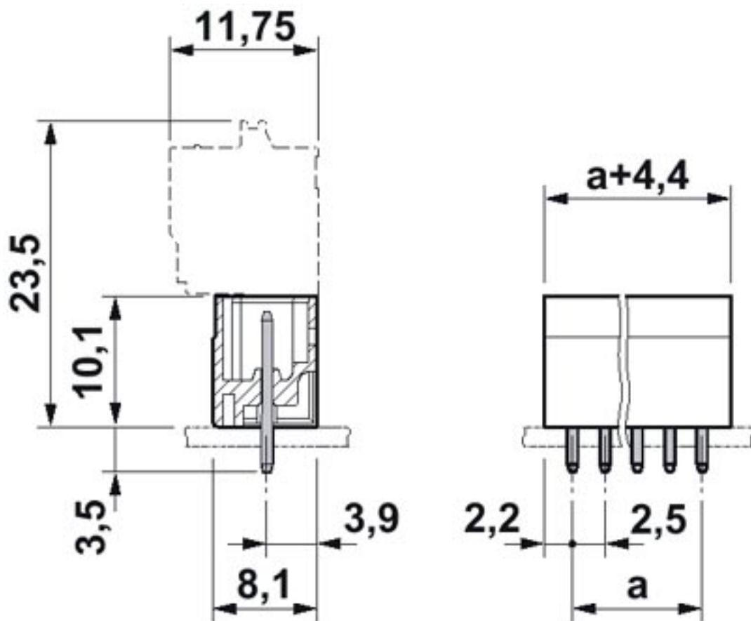
外形寸法
