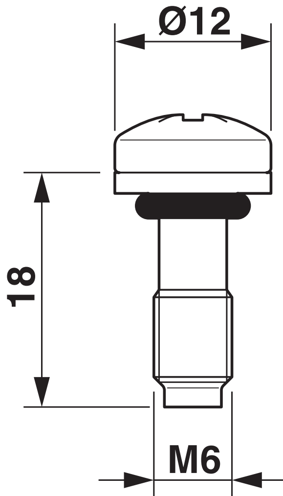
尺寸图
