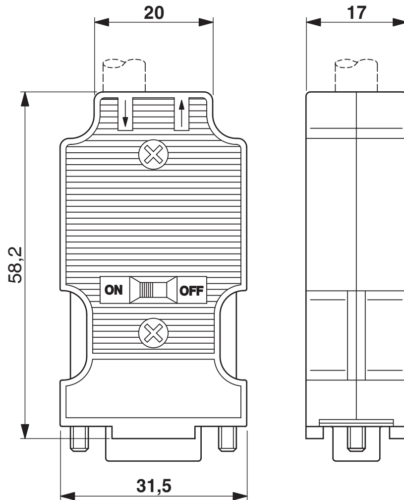
Maßzeichnung
