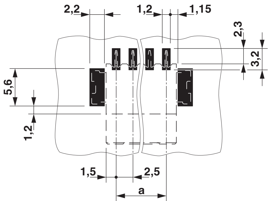
开孔图/焊盘环宽
