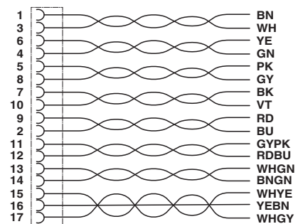
回路図
