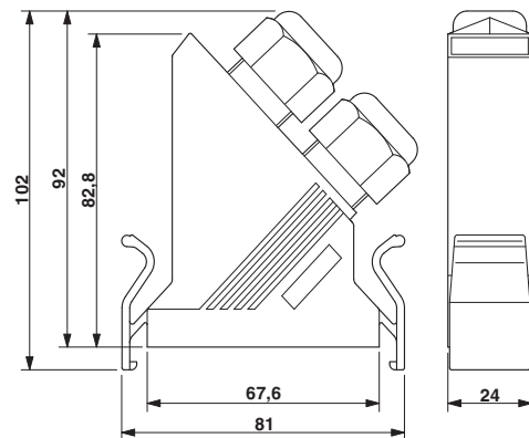
Dessin coté
