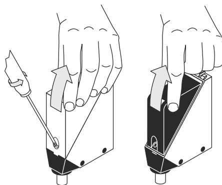
Figura 2: Aprire il sensore
