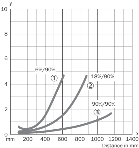
插图 6: WT34-Xx4x, -Xx5x, 红光
