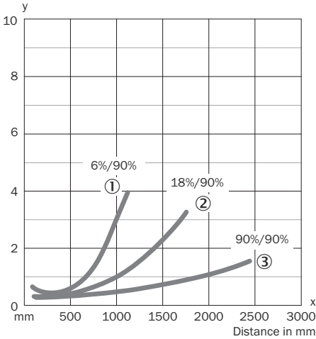
Rysunek 7: WT34-Xx1x, -Xx2x, światło podczerwone
