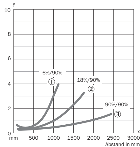
Abbildung 7: WT34-Xx1x, -Xx2x, Infrarotlicht
