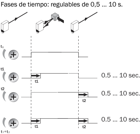
Figura 8: Funciones de temporización
