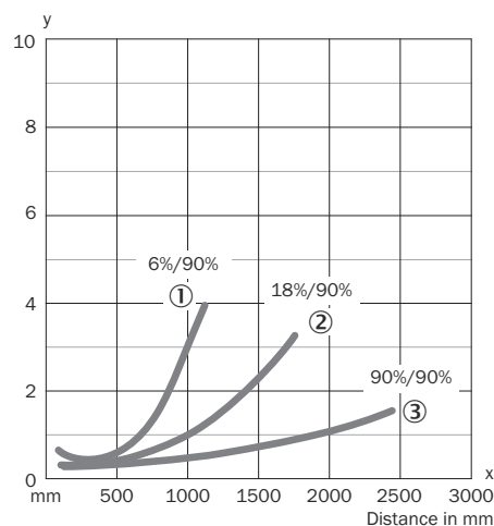
図 7: WT34-Xx1x, -Xx2x, 赤外光
