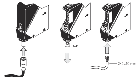
Illustration 3: Raccordement électrique
