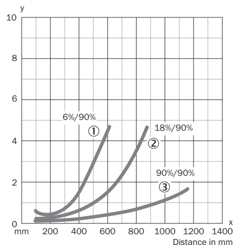
Рисунок 6: WT34-Xx4x, -Xx5x, красный свет
