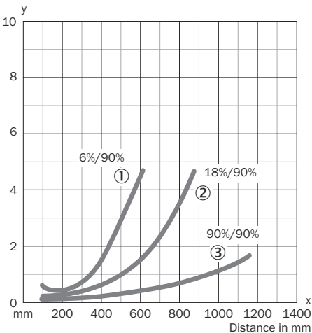
Figura 6: WT34-Xx4x, -Xx5x, luz vermelha
