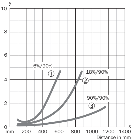
Rysunek 6: WT34-Xx4x, -Xx5x, światło czerwone
