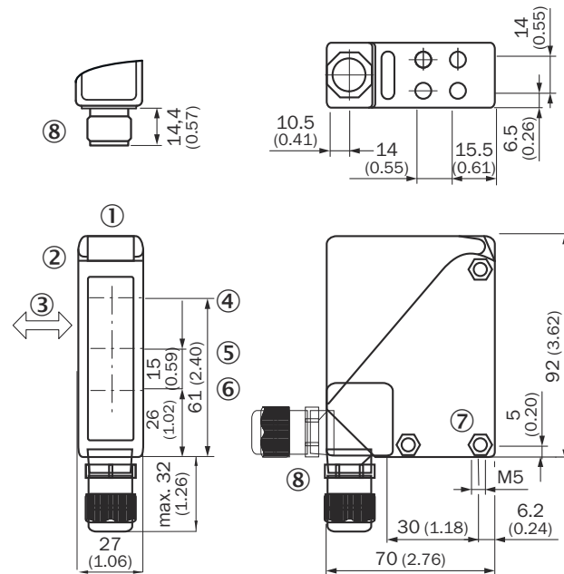
Abbildung 9: Maßzeichnung
