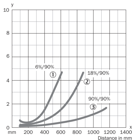
図 6: WT34-Xx4x, -Xx5x, 赤色光
