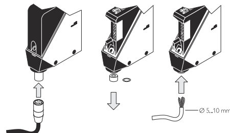
Figura 3: Collegamento elettrico
