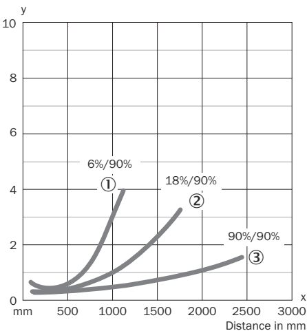
插图 7: WT34-Xx1x, -Xx2x, 红外线
