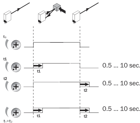
Rysunek 8: Funkcje czasu
