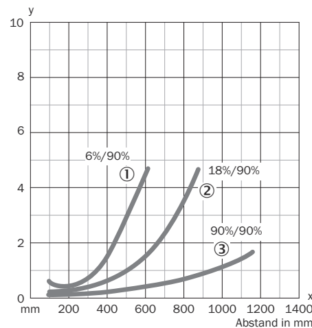
Abbildung 6: WT34-Xx4x, -Xx5x, Rotlicht
