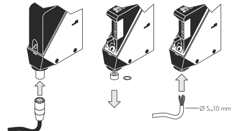
Figura 3: Conexión eléctrica
