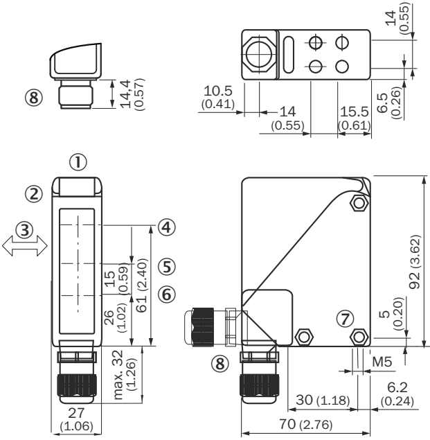
插图 9: 尺寸图
