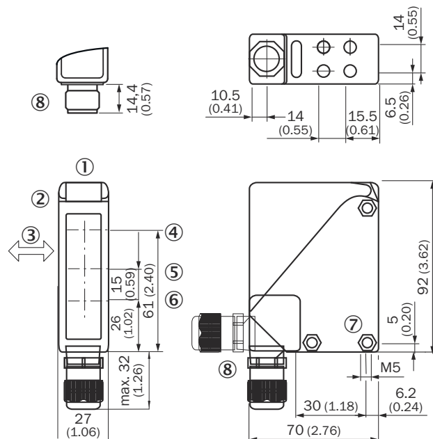
Figura 9: Desenho dimensional
