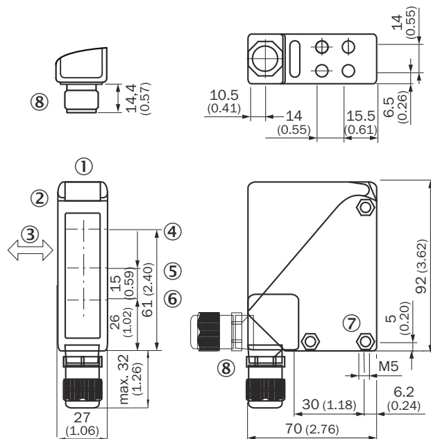
Рисунок 9: Масштабный чертёж
