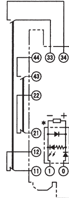
G7SA-2A2B montado
