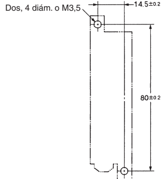
G7SA-5A1B montado
