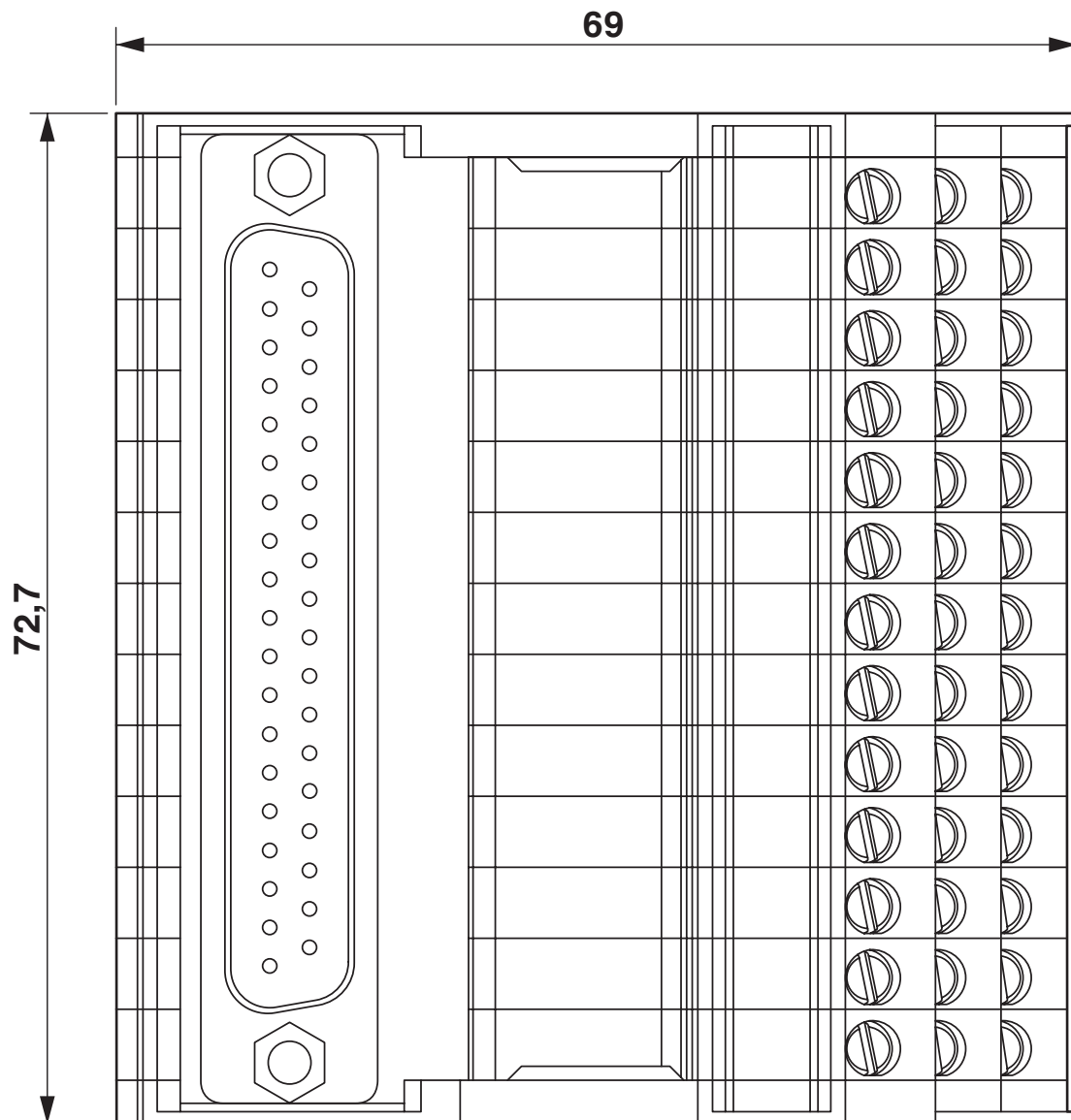
Maßzeichnung
