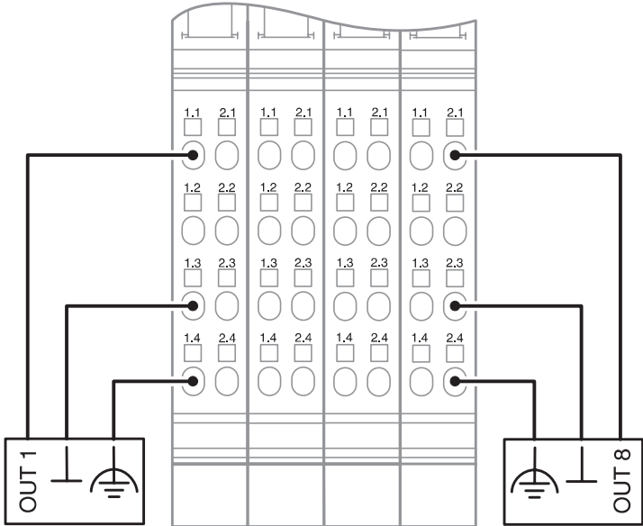
接线图
