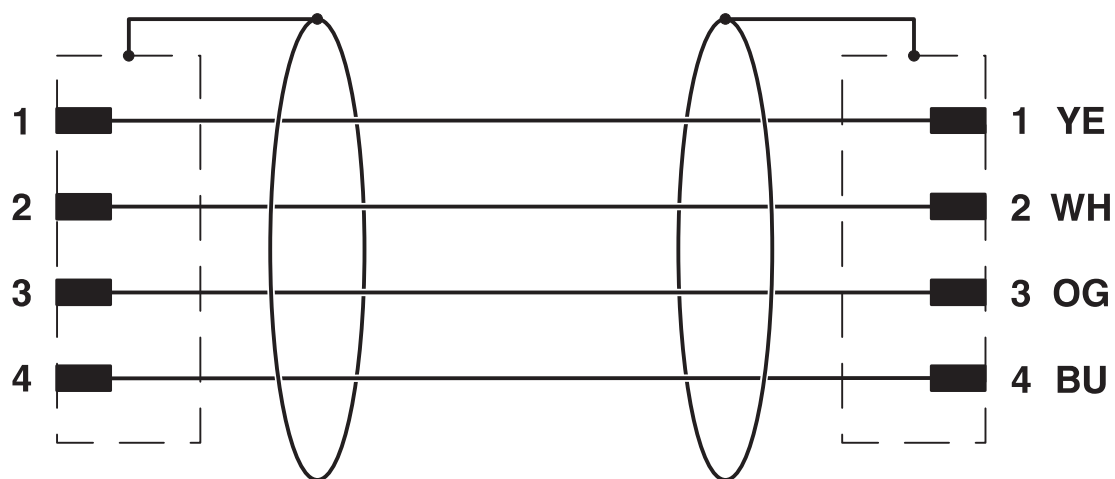
电路图
