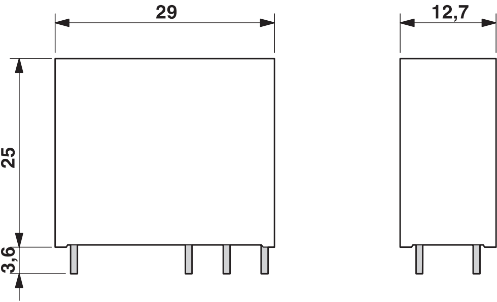
尺寸图
