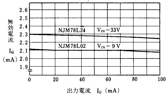
NJM78L02 / L24 負荷時無効電流特性例
