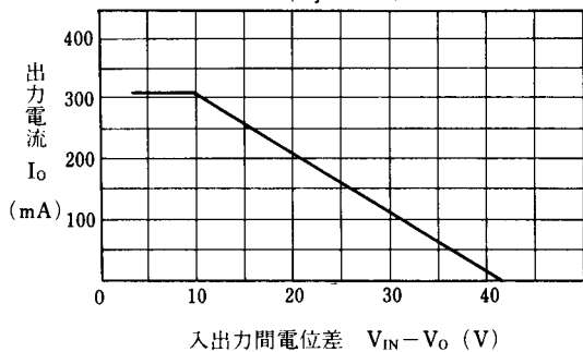
NJM78L00 シリーズ保護回路動作特性例
