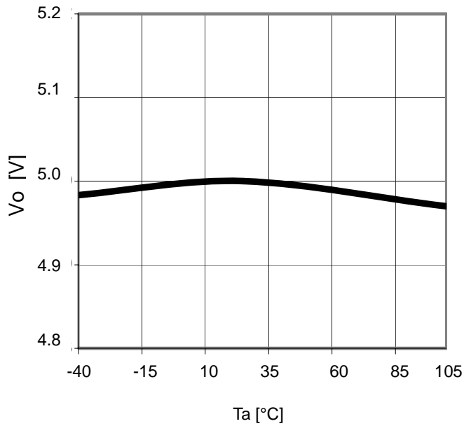
Fig.21 Ta-Vo (Io=0mA)
